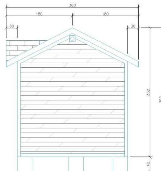
外觀尺寸圖
